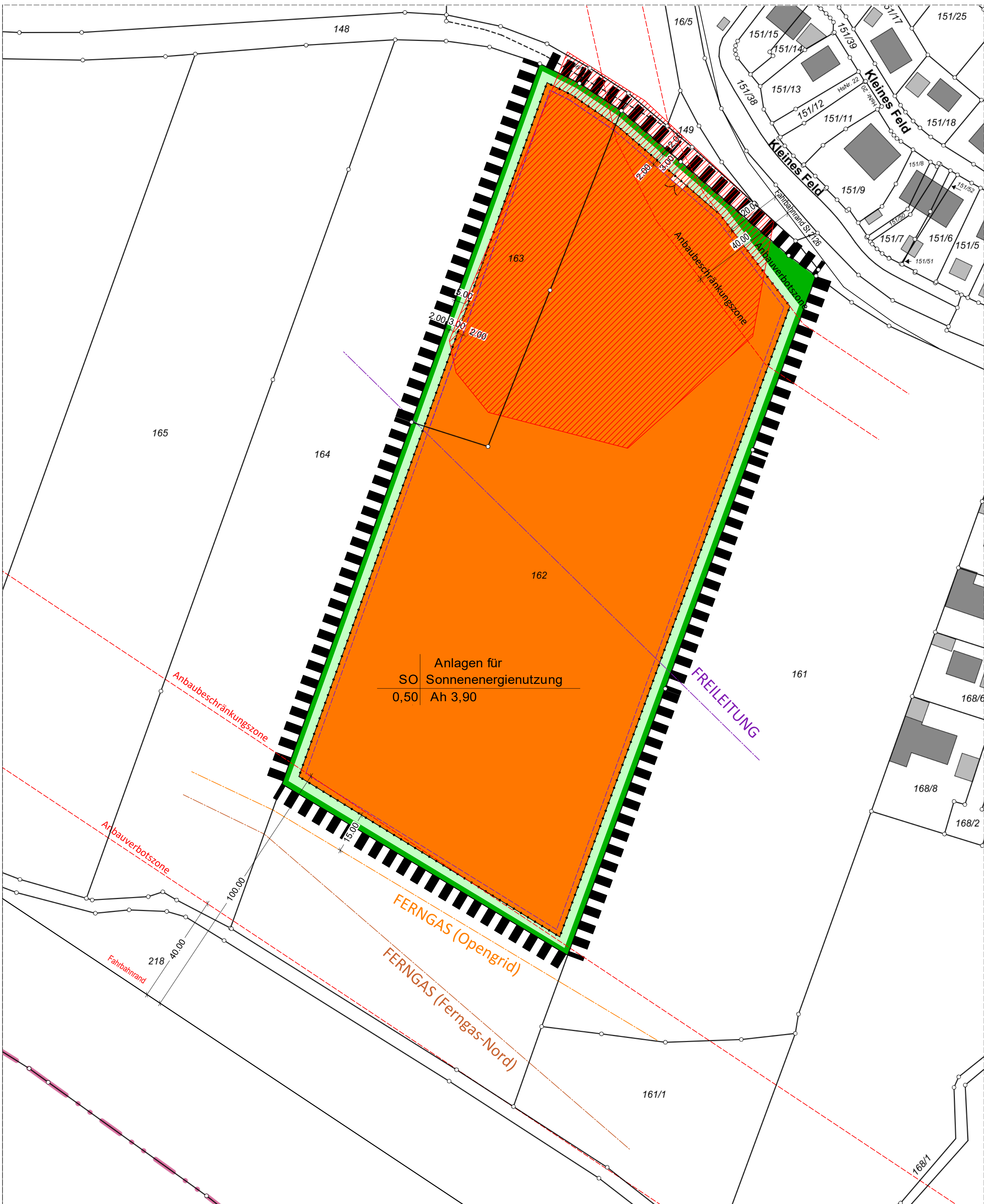
Lageplanausschnitt Solarpark (Flur Nr. 162, Gmrg. Schwanenkirchen)
